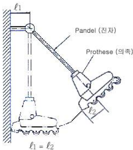
그림 3-1 제동장치의 수평 충돌시험
