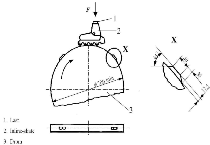
그림 5 주행시험
