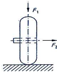
그림 1 마찰저항시험
