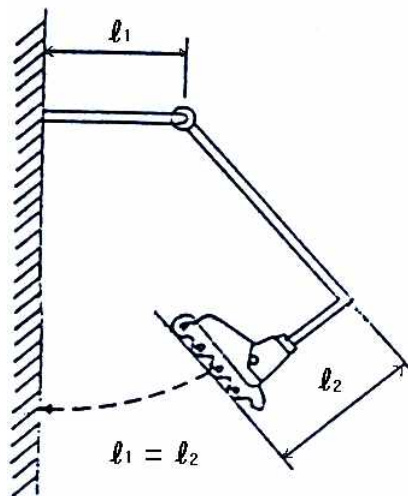
그림 4 수직 충돌시험
