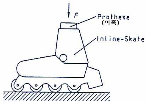
그림 7 압축하중시험
