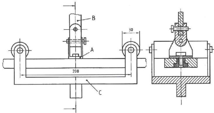
<그림 8> 당김 장치가 부착된 만능재료 시험기
