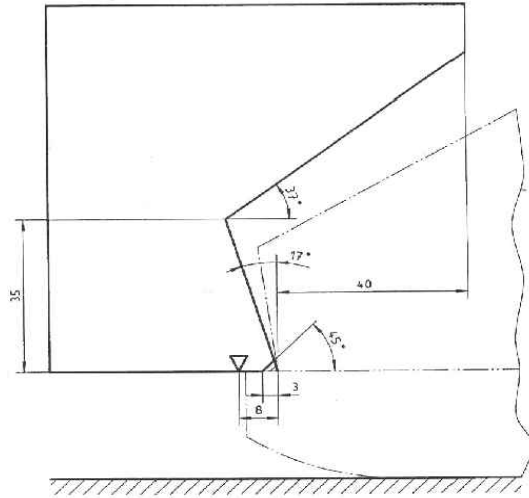
<그림 4> 부츠 발끝에 대한 시험의 예(최대형상)
