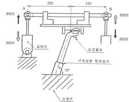
부속서 3 그림 1 시트 포스트의 강도
