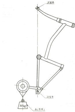
그림 12 후방하중 시험
