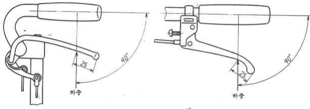
그림 4 수동 브레이크 레버에 가하는 하중의 위치 및 방향
