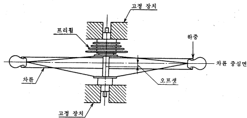
그림 10 차륜의 정하중 시험
