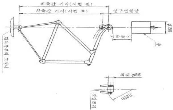
부속서 1 그림 4 차체 하중낙하 충격시험
