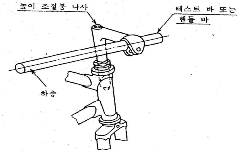
그림 7 핸들 스템과 포크 스템의 고정 시험
