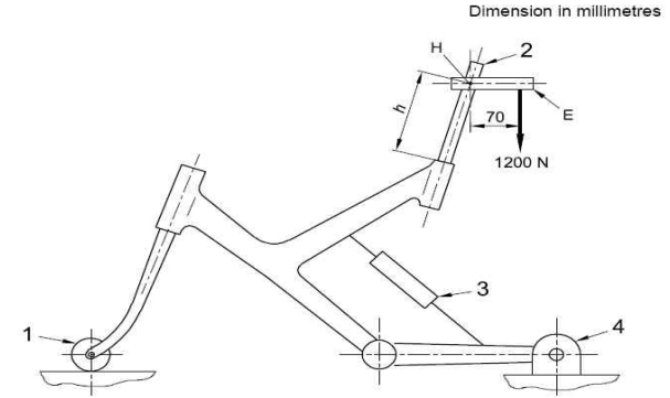
부속서1 그림 2 수직하중 피로시험
