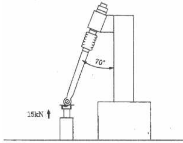
부속서 2 그림 3 수직 부하 시험
