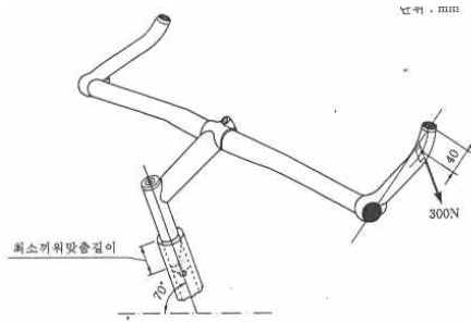
부속서 5 그림 1 바 엔드 바의 고정강도
