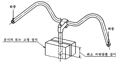
그림 8 핸들 바와 스템의 고정시험
