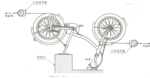
그림 6 수동 브레이크의 제동력 시험
