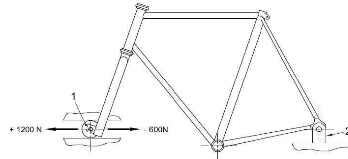
부속서1 그림 3 수평하중 피로시험
