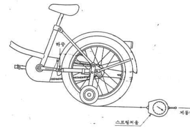
그림 7 코스터 허브의 제동력 시험
