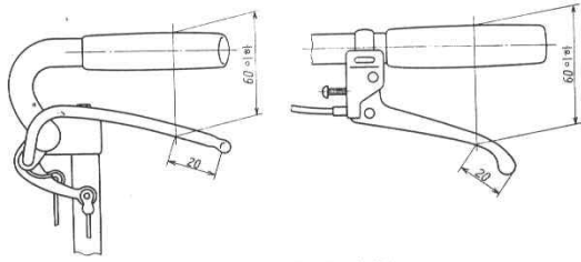
그림 1 브레이크 레버의 벌림
