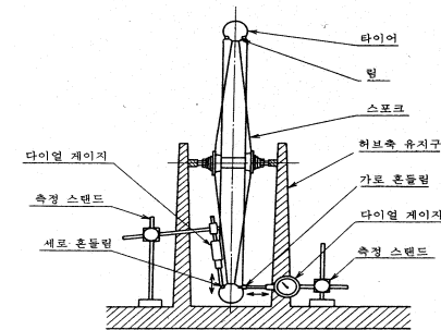
그림 2 바퀴 회전 정밀도 측정방법
