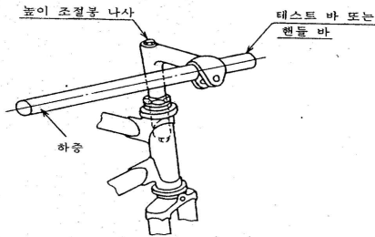
그림 9 핸들 스템과 포크 스템의 고정시험
