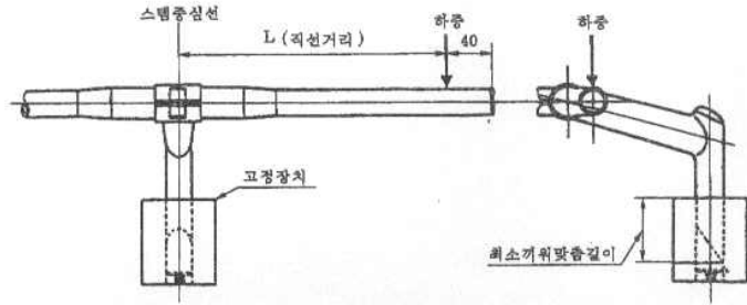
부속서 4 그림 1 한쪽 하중시험
