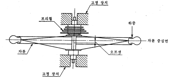
그림 1 바퀴의 정하중 시험
