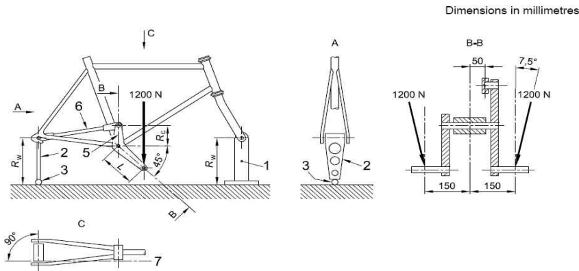
부속서1 그림 1 페달력을 인가한 프레임 피로시험
