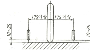
그림 3 뒷차륜과 좌우 보조차륜의 고저차
