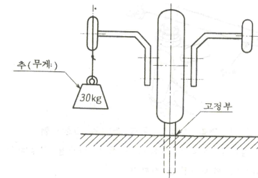
그림 11 수직하중 시험
