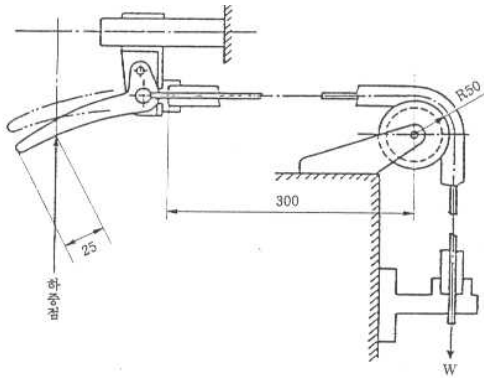
부속서 8 그림 1 브레이크 와이어의 반복 강도 시험
