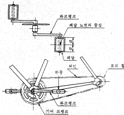
그림 5 코스터 허브 부착 유아용 자전거의 하중 시험
