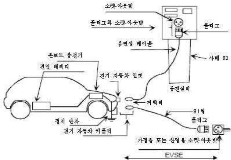
그림 1 - "A형" 연결
