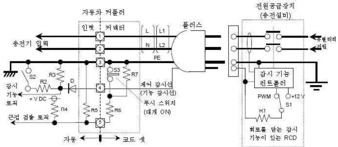
그림 B.3 - 기본 단상 자동차 커플러를 사용한 모드 3의 B형
