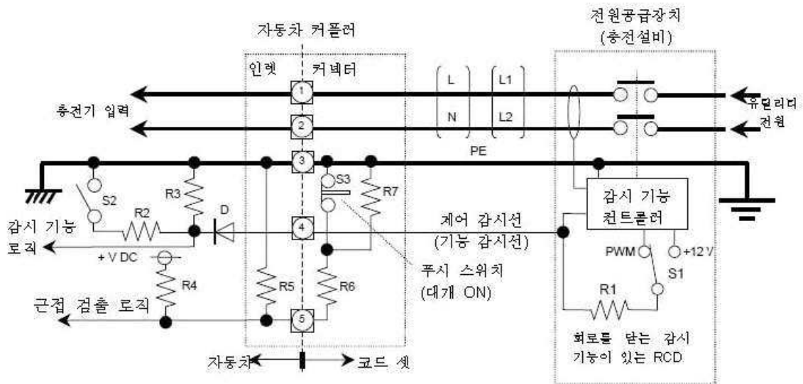
그림 B.4 - 기본 단상 자동차 커플러를 사용한 모드 3의 C형
