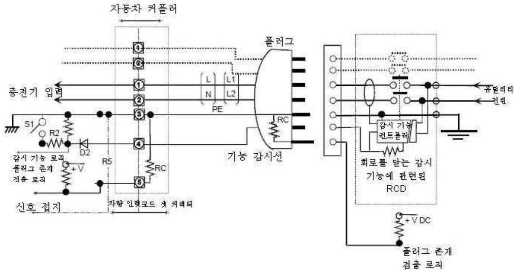
그림 B.5 - 근접 푸시버튼 스위치 S3이 없는 기본 단상 자동차 커넥터를 사용한 모드 3의 B형
