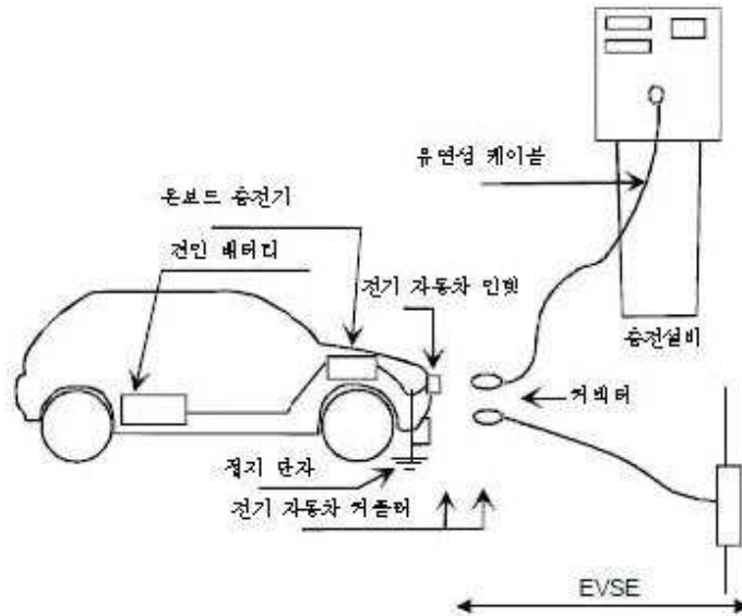
그림 3 - "C형" 연결
