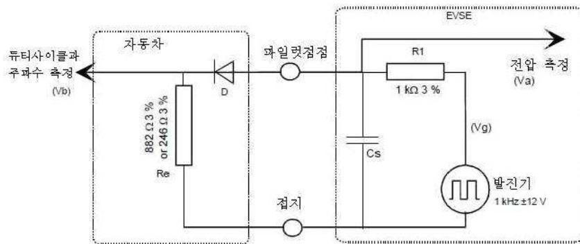
그림 A.2 - 간이 제어 파일럿 회로
