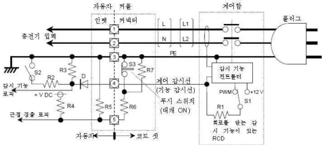
그림 B.2 - 기본 단상 자동차 커플러를 사용한 모드 2의 B형
