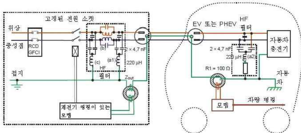
그림 C.1 - 보조선이 없는 파일럿 기능의 예
