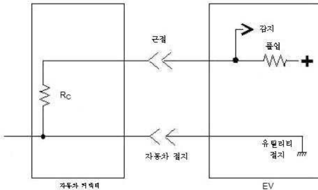
그림 B.6 - 케이블 어셈블리의 전류 용량 부호화에 대한 다이어그램
