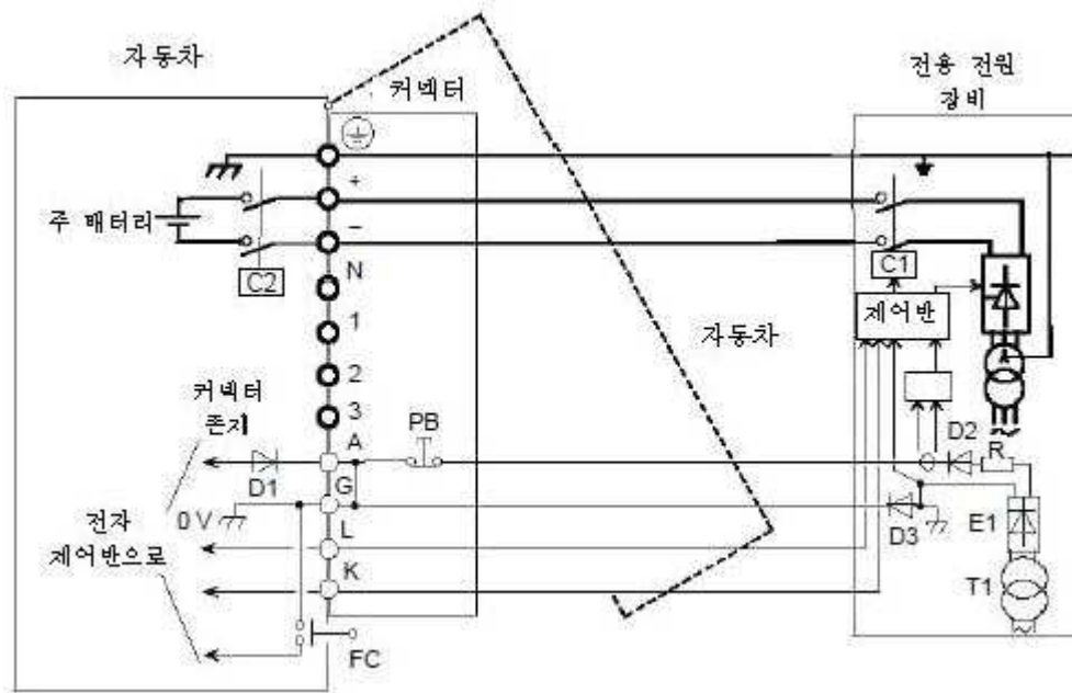
그림 B.7 - 범용 자동차 커플러를 사용한 모드 4의 C형
