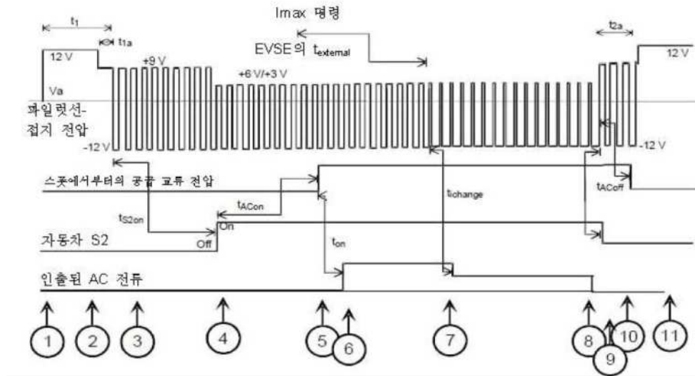
그림 A.3 - 통상적인 동작 상태에서의 전형적인 충전 사이클
