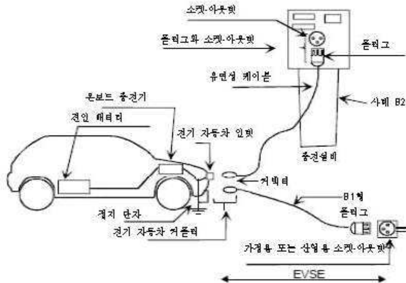
그림 1 - "A형" 연결
