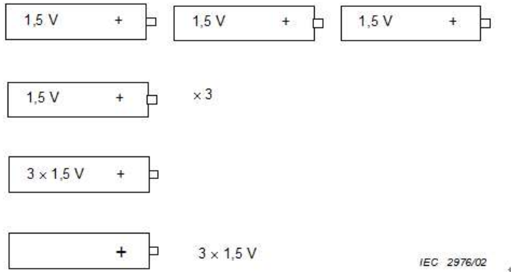
그림 S.1 3개의 배터리를 나타내는 표현 방법
