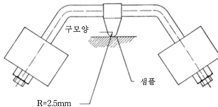
그림 1 - 볼-프레셔 시험장치
