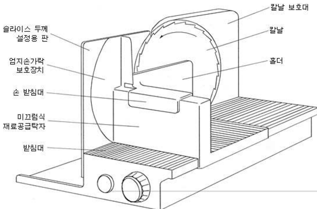
그림 101 - 슬라이스기
