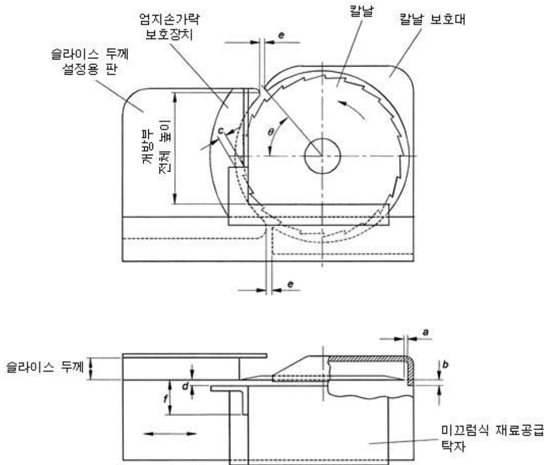
그림 102 - 슬라이스기의 보호장치
