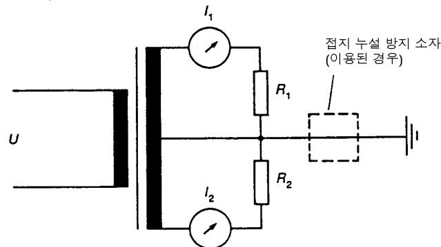
그림 C.1 정상 부하 등가 저항(중성점 접지 변압기에 대한 예)
