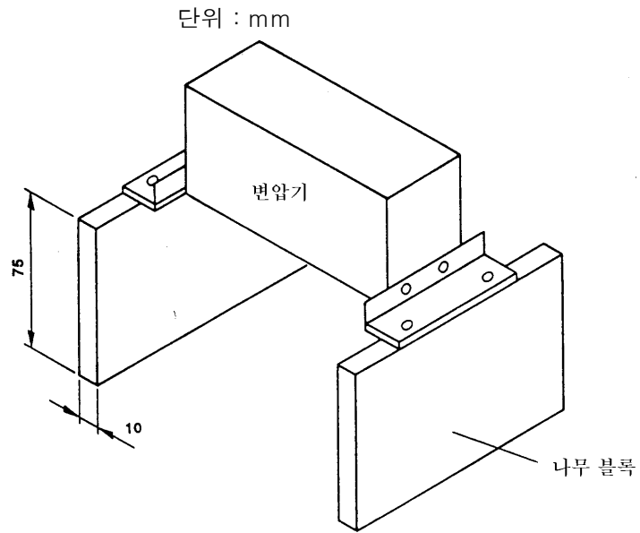
그림 C.2 온도 상승 시험을 위한 시험 배열
