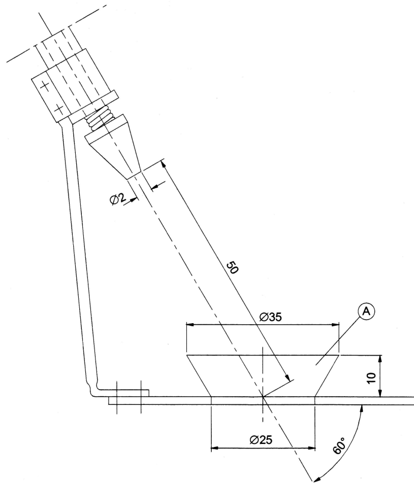
그림 101 물 튀김 장치
