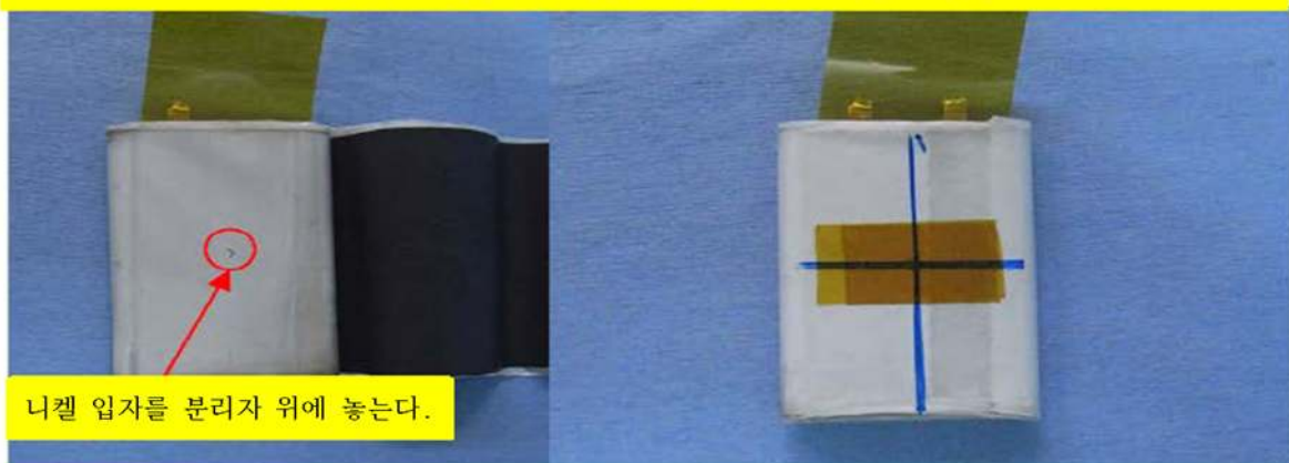
그림 A.8 — 각형 단전지 해체
