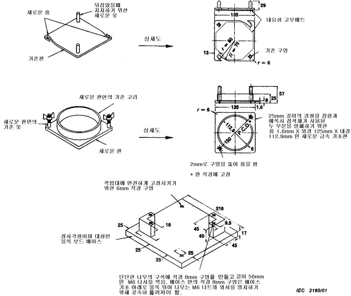
그림 2b - 상세도 (Cobb 흡수 시험기에 필요한 변형)
