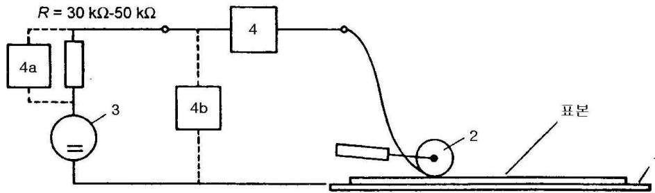
그림 3 - 전도 입자용 시험 기구의 도식적인 배치
